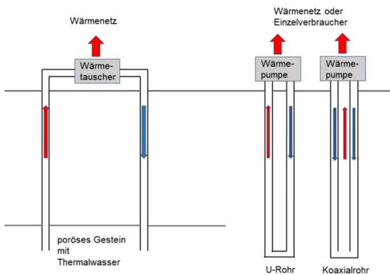
Abbildung 4-8: Technische Lösungen zur geothermischen Energiegewinnung: links offenes System mit Nutzung von Thermalwasser, rechts geschlossene Systeme mit U- und Koaxialrohr.
