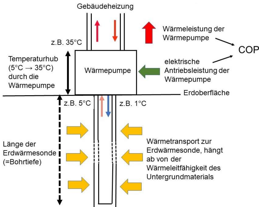
Abbildung 4-12: Arbeitsweise einer Wärmepumpe zur Erreichung der erforderlichen Heiztemperatur.
