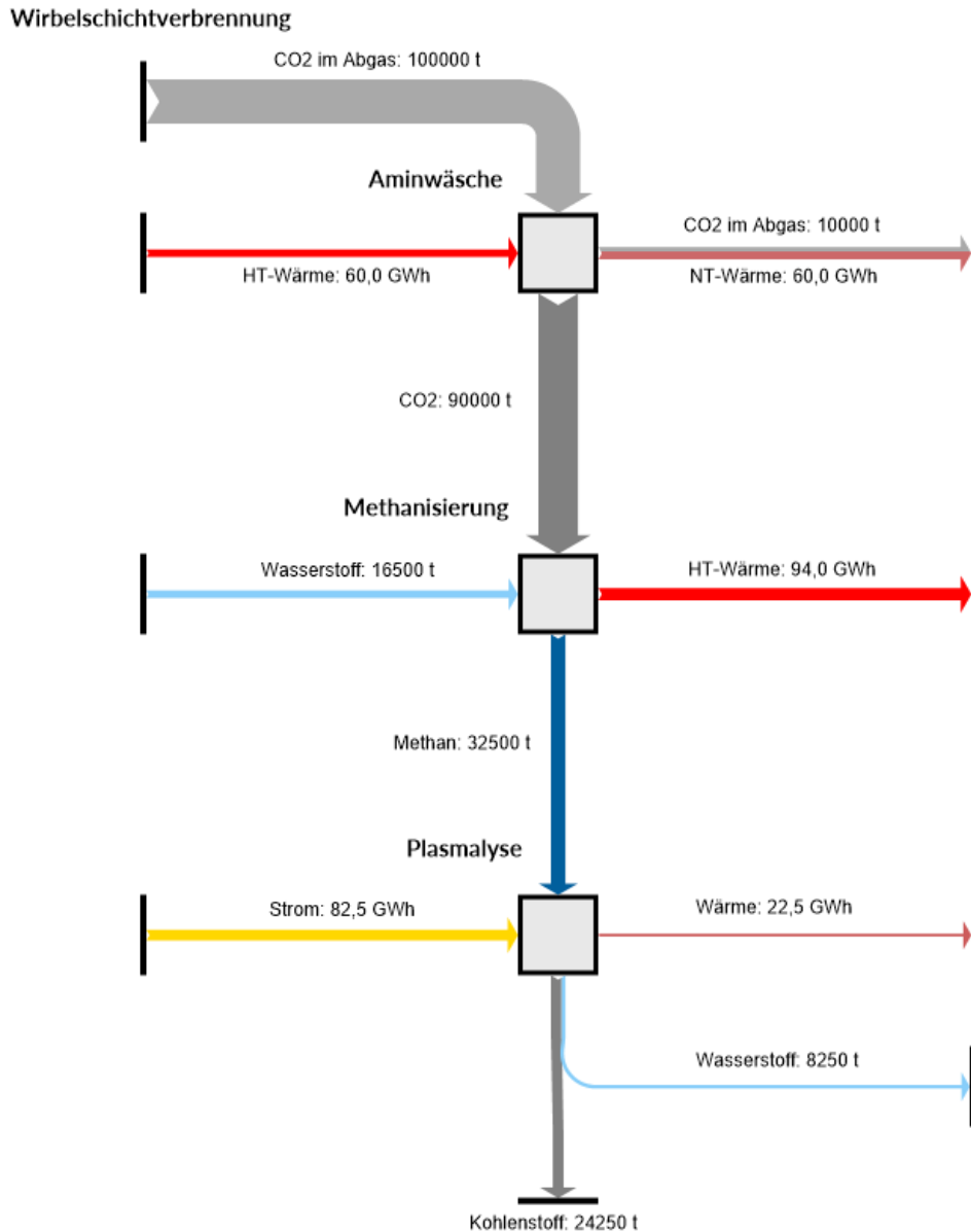
Abbildung 4-27: Detaillierte Prozesskette TEV CCU
