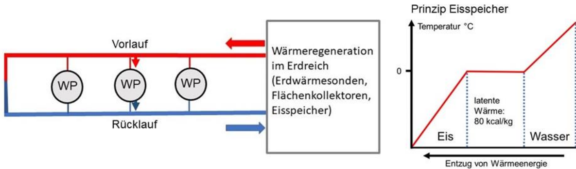
Abbildung 4-16: Prinzip kaltes Nahwärmenetz und Erdeisspeicher
