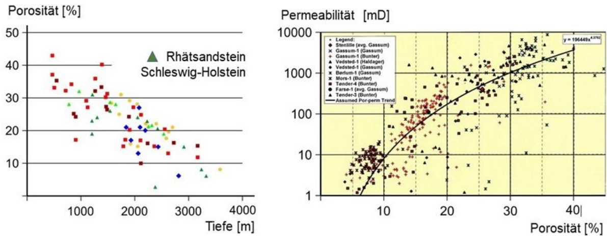
Abbildung 4-22: Links: Porositäts-Tiefenrelation für Reservoirsandsteine aus Dänemark und Norddeutschland (Thomsen 2013), rechts: Porositäts-Permeabilitätsrelation für Reservoirsandsteine aus Dänemark (Mathiesen et al. 2011)
