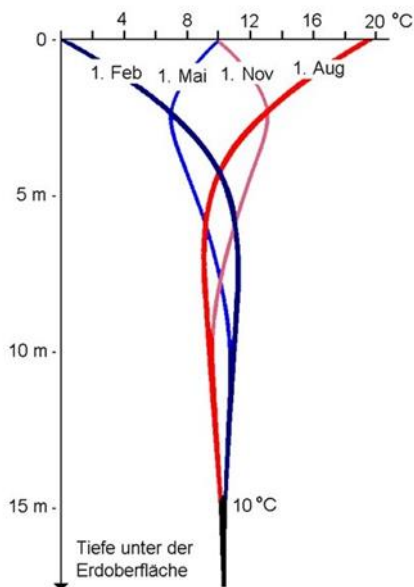
Abbildung 4-10: Temperatur-Tiefenprofil für den oberflächennahen Bereich
