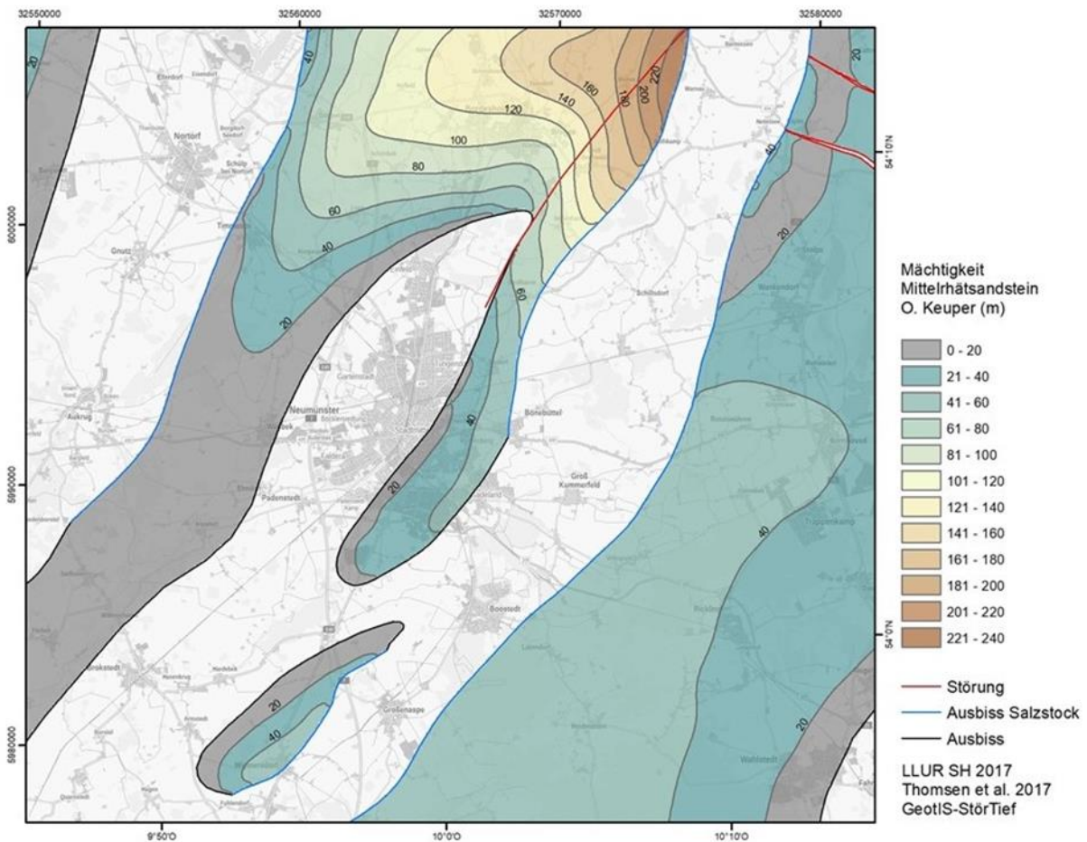
Abbildung 4-21: Mächtigkeit des Mittelrhätsandsteins im oberen Keuper im Raum Neumünster (LLUR 2022)
