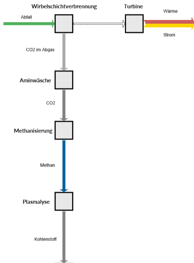
Abbildung 4-26: Prozesskette TEV CCU
