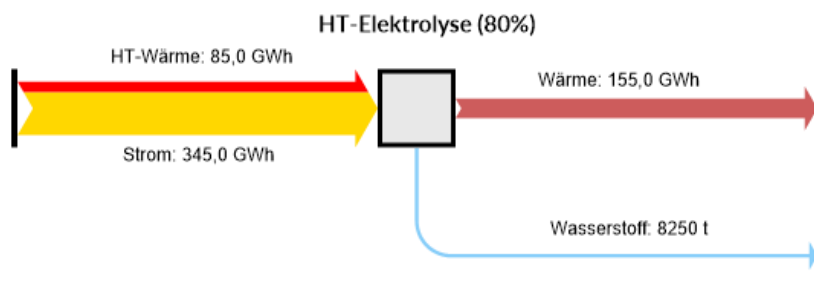
Abbildung 4-28: Erweiterter Prozess TEV CCU
