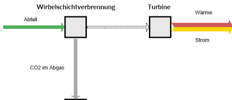
Abbildung 4-25: Prinzipschema der TEV Neumünster ohne Qualifizierung der Ströme
