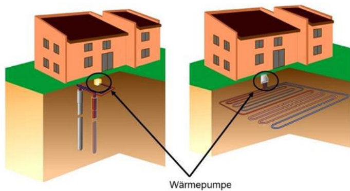
Abbildung 4-11: Erdwärmesonde (a) und Erdwärmekollektor (b). Die Wärmegewinnung aus dem Untergrund erfolgt über eine zirkulierende Wärmeträgerflüssigkeit in den Sonden- und Kollektorrohren.
