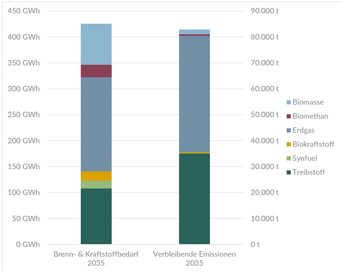
Abbildung 6-7: Brenn- & Kraftstoffbedarf und verbleibende Emissionen 2035
