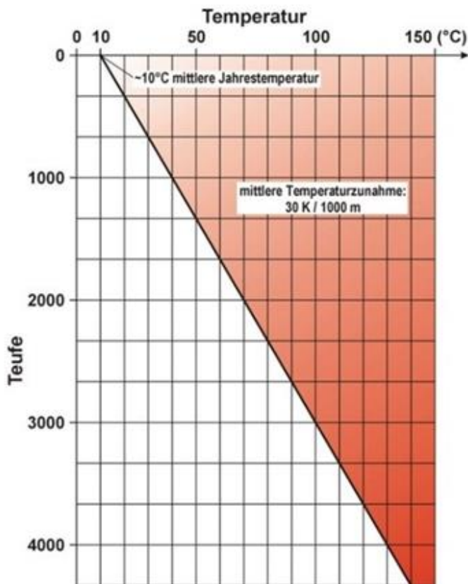
Abbildung 4-7: Zunahme der Temperatur mit der Tiefe
