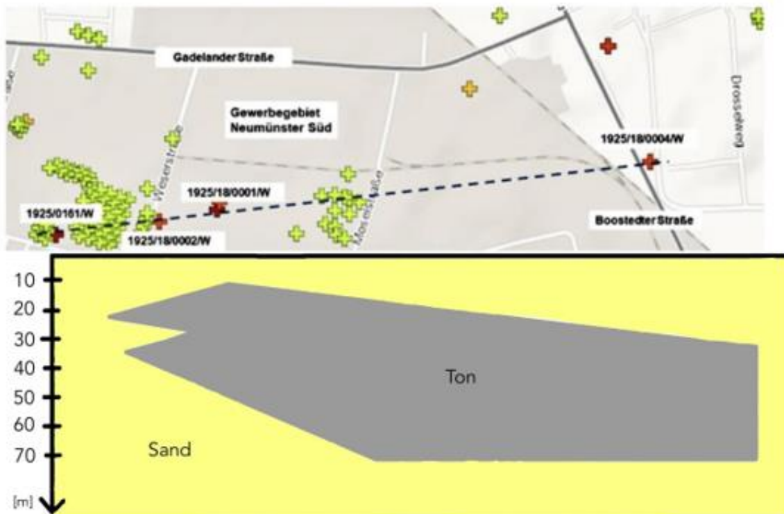
Abbildung 4-15: Schnitt durch eine Tonlage im Gewerbegebiet Neumünster Süd. (Kartengrundlage BGR Bohrpunktkarte, Bohrinformation LLUR)
