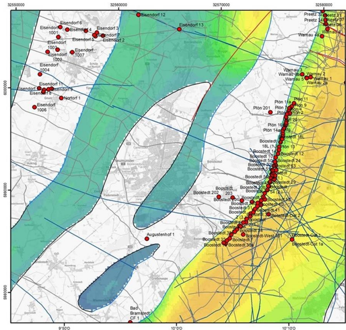
Abbildung 4-18: Tiefbohrungen und seismische Messprofile im Raum Neumünster, farbkodiert ist die Basis-tiefe des oberen Keupers (=Rhät) (LLUR 2022).
