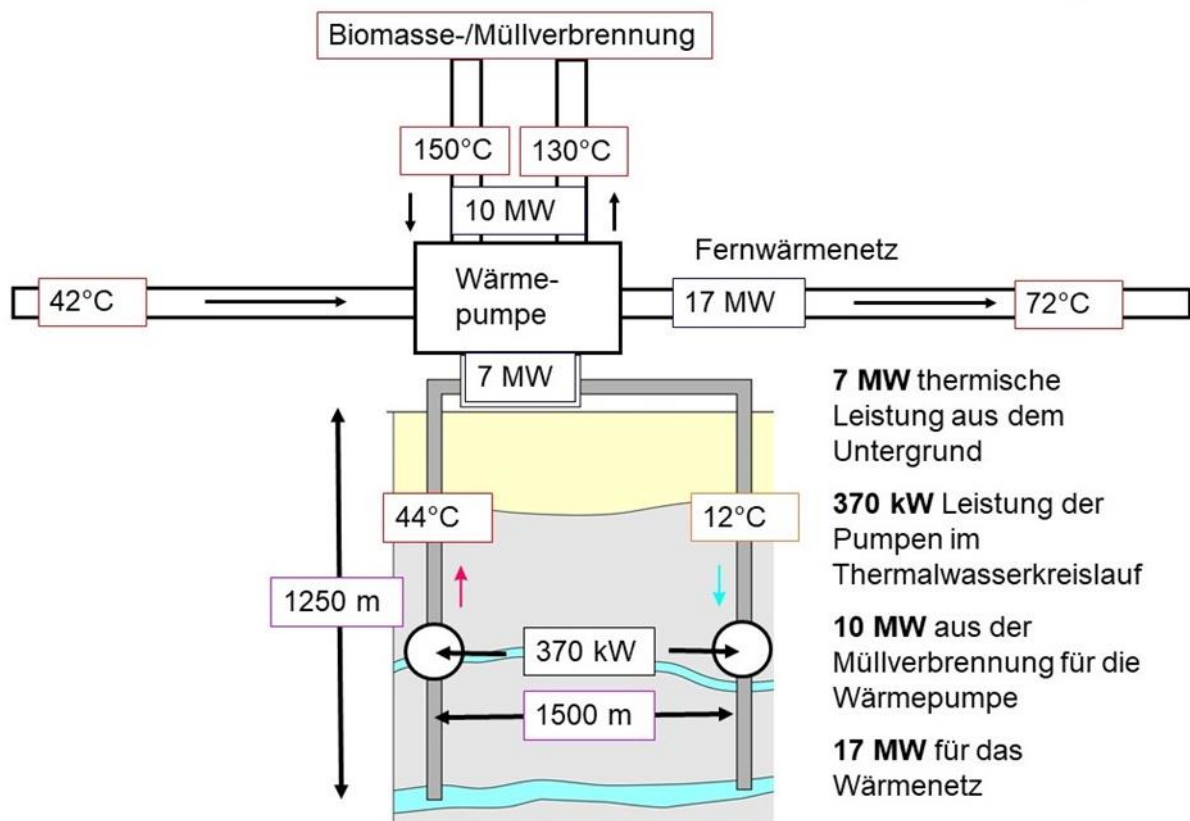
Abbildung 4-23: Schematische Funktionsweise des Heizkraftwerks Thisted (DK).
