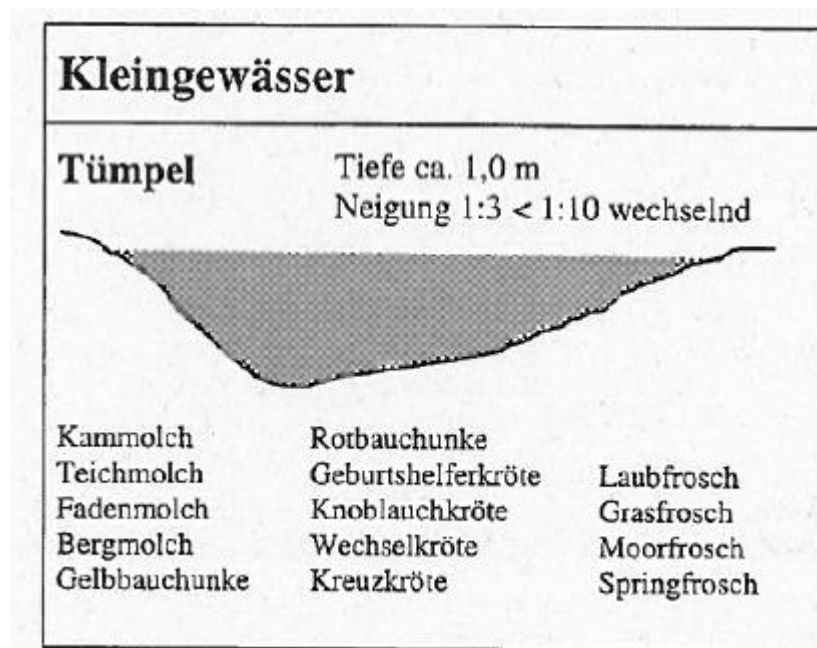
Bild 8: Beispielzeichnung (unmaßstäblich) zur Anlage eines Laichgewässers. Typ Tümpel, ca. 500 m 2 . Form und Gestalt sind den örtlichen Gegebenheiten anzupassen.
