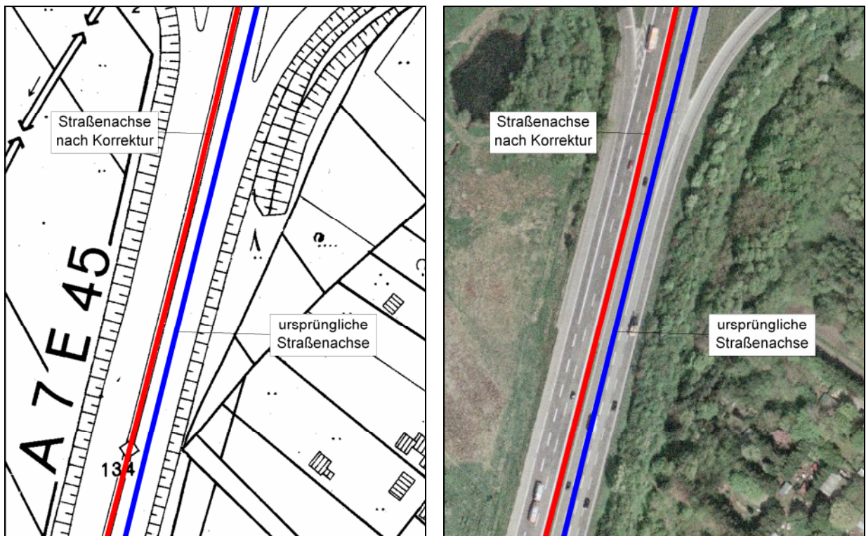
Abbildung 2: Lagekorrektur Straßenachsen (A7 südlich AS Quickborn), M 1:2.500
