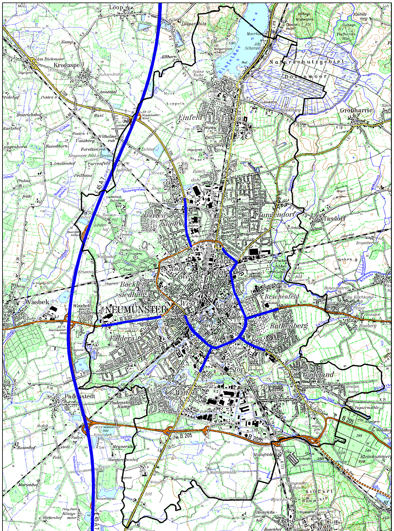
Abbildung 3: untersuchtes Straßennetz, M 1: 67.000
